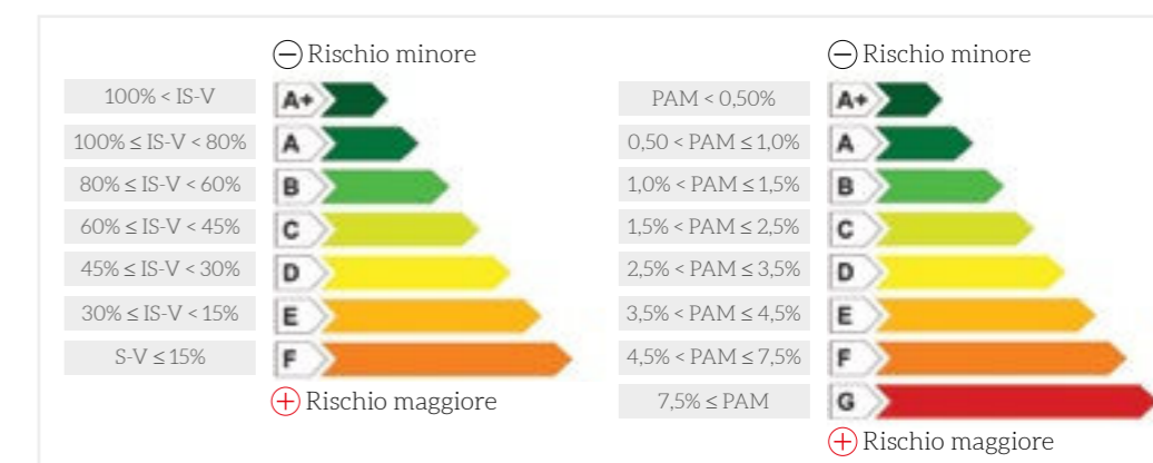
Esempi di classificazione sismica degli edifici Articolo 3 del D.M. 7/3/2017 n°65
